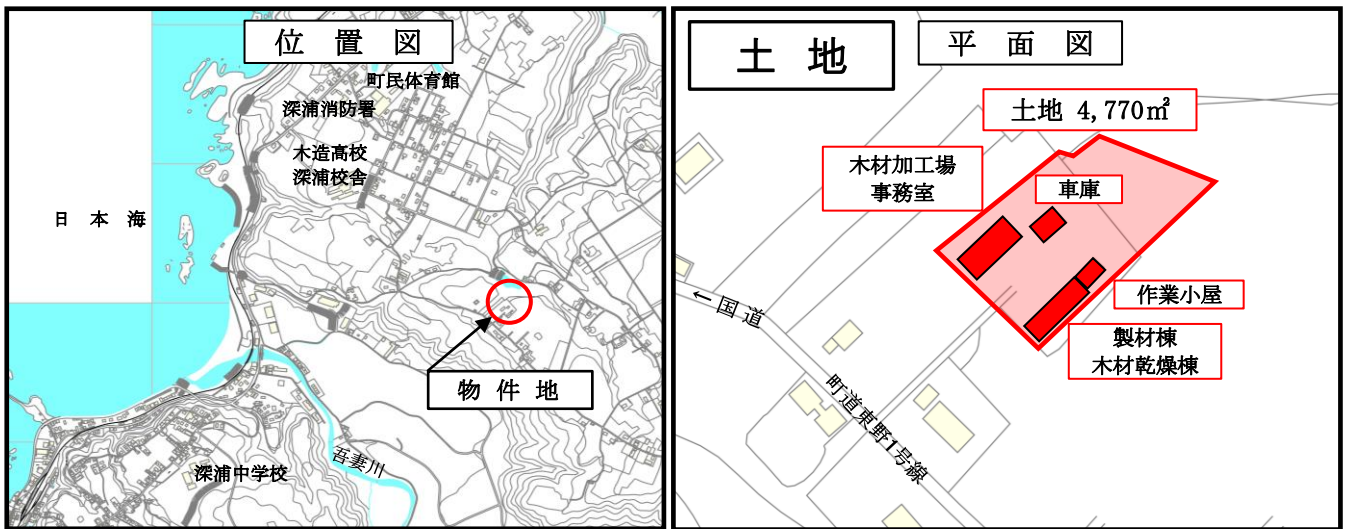
木材加工場・事務室（木造平屋建）454.78㎡
