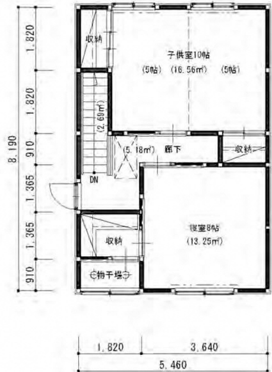
2 階間取り
