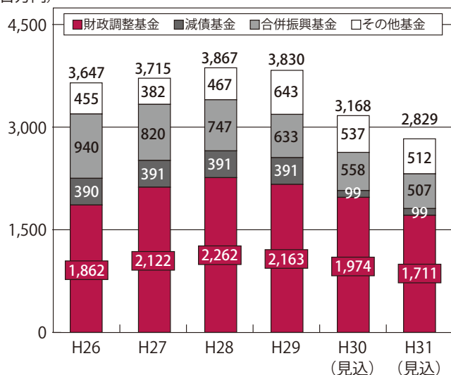
(百万円) 基金（一般会計）の推移(平成31年度見込みまで)
